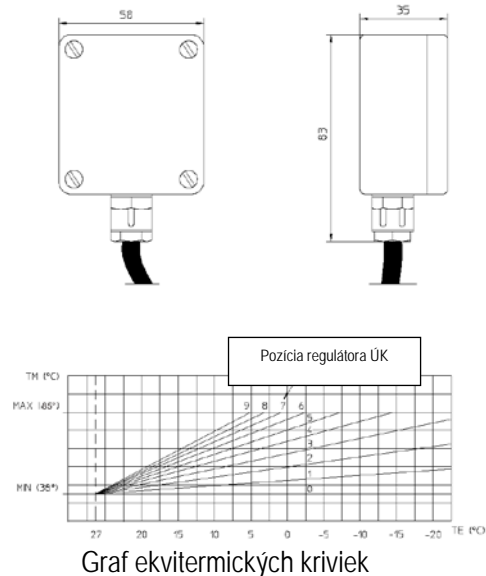
Snímač vonkajšej teploty
