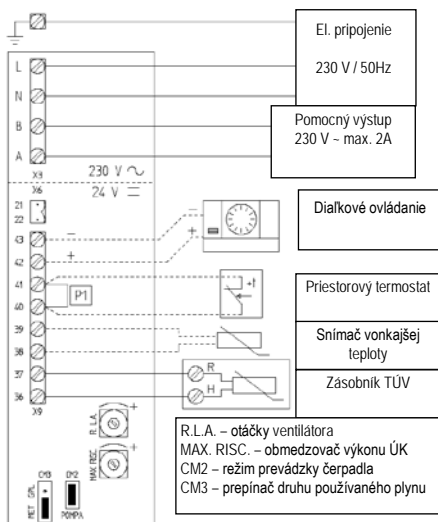
Svorkovnica kotla
