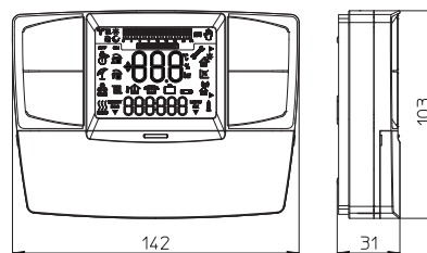
Ovládanie Vzdialený Priateľ V2 (CAR V2 )
