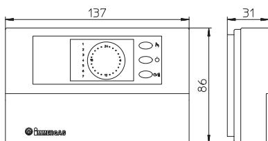
Digitálny časový termostat On/Off
