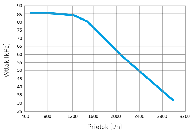
Graf obehového čerpadla pre MAGIS M12 T EH9/14 T EH9/16 T EH9 užitočný výtlak pre systém ÚK
