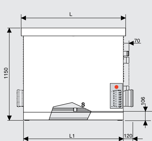
(●) ARES 200 - 300 Tec ErP hrdlo vnútri plášťa
