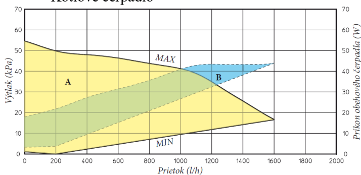
Kotlové čerpadlo
