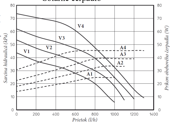
Solárne čerpadlo
