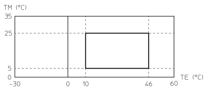
Prevádzkové limity tepelného čerpadla v režime chladenia
