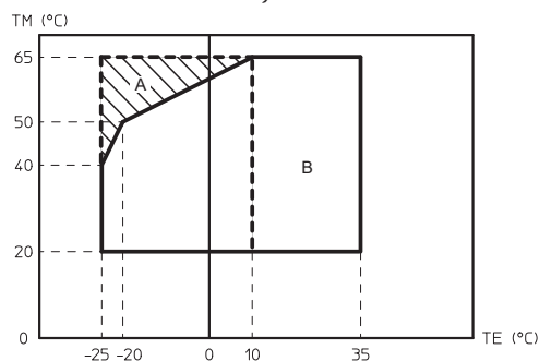
Prevádzkové limity tepelného čerpadla v režime vykurovania
