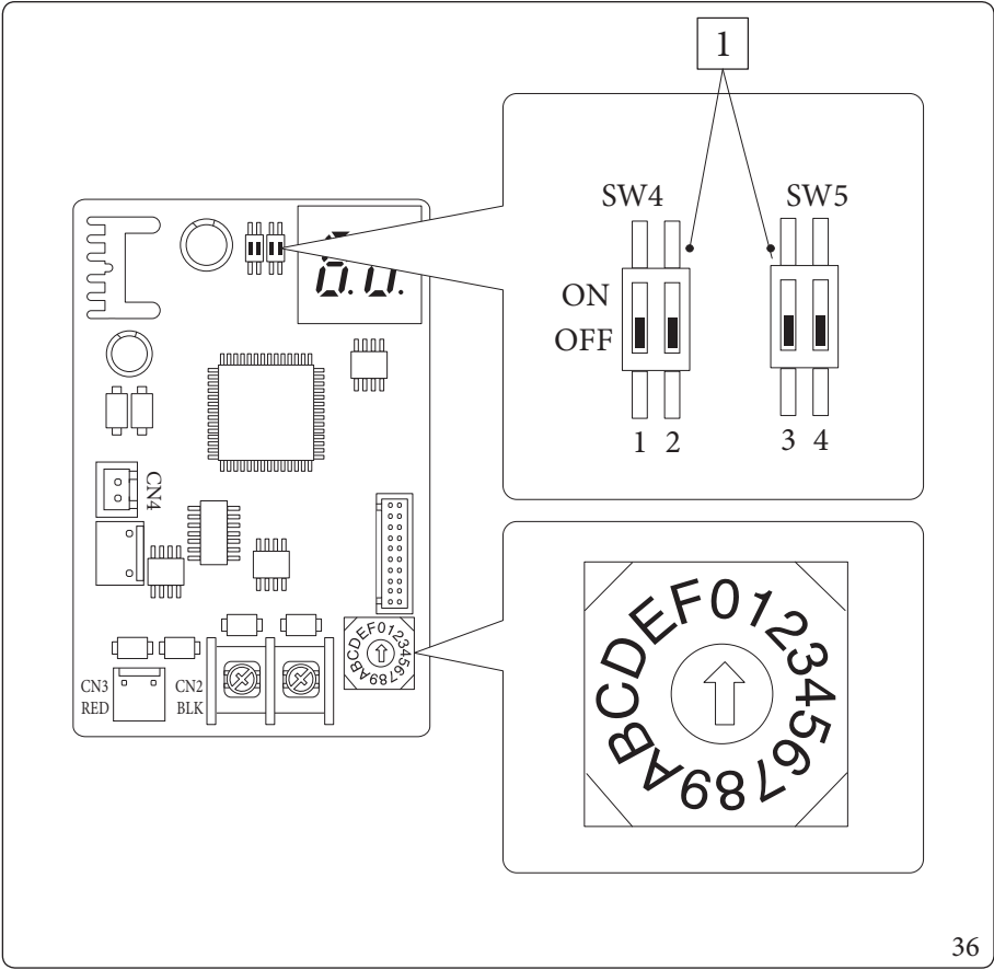
Legenda (Obr. 36): 1 - Továrenské nastavenia: nemeniť
