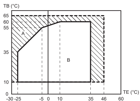
Prevádzkové limity v režime TUV
