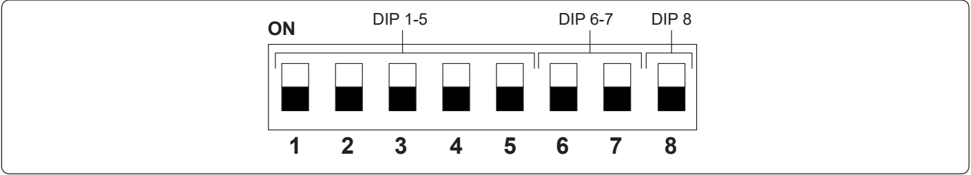
Konfiguračná tabuľka DIP-Switch
